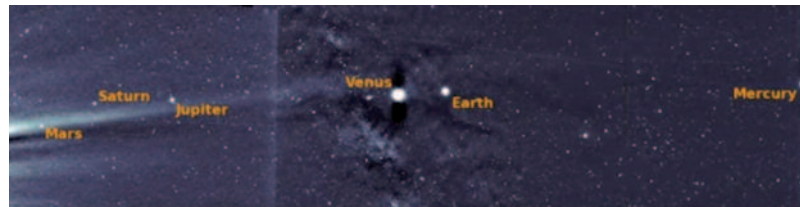
Sei pianeti visti dalla sonda Solar della NASA
