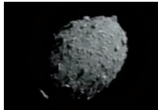
Dimorphos ripreso da LiciaCube pochi istanti prima di essere colpito da Dart
