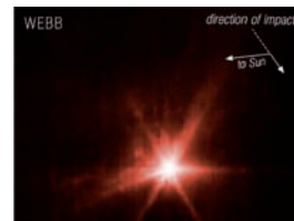
Riprese da Webb dopo l'impatto
