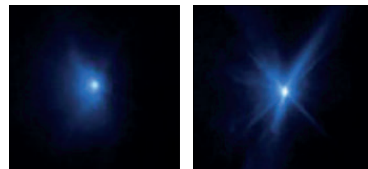
Riprese da Hubble 22 minuti e otto ore dopo l'impatto
