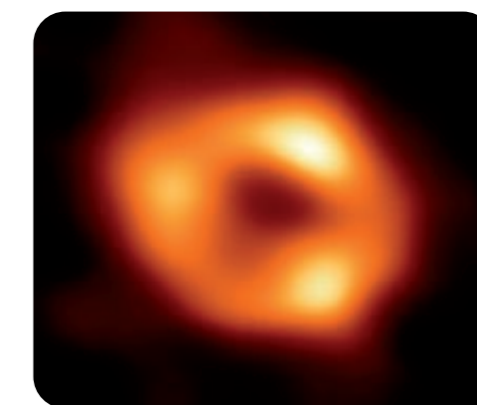
È stata catturata dall'Event Horizon Telescope (EHT), un array che collega otto radio osservatori esistenti in tutto il pianeta per formare un unico telescopio virtuale delle dimensioni della Terra. La foto è stata pubblicata il 12 maggio 2022.
